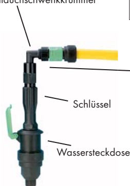
Schlauchschenkrümmer
